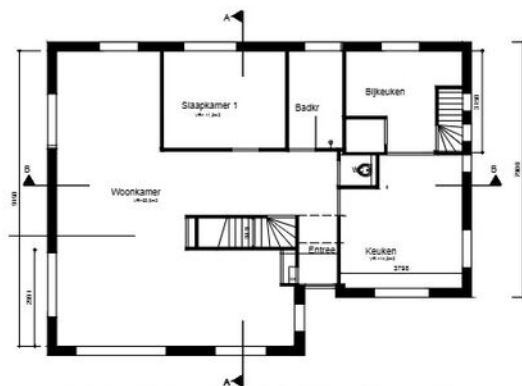
WOONVERDIEPING-BEGGR GO = 102m 2
