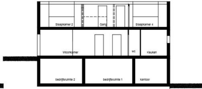
DOORSNEDE B-B
