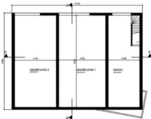
BEDRIJFSRUIMTE GO = 113m 2
