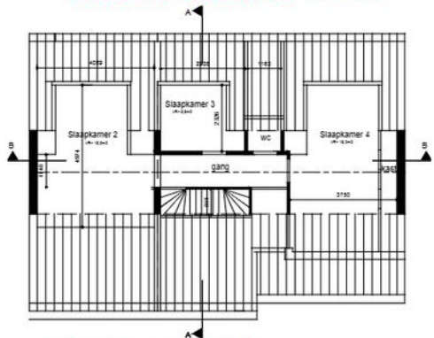
DAKVERDIEPING GO = 48m 2
